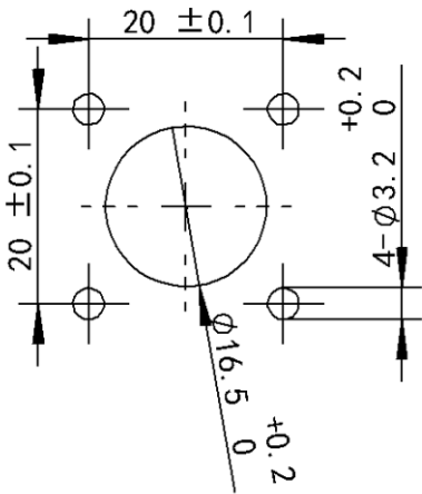
安装开孔图
